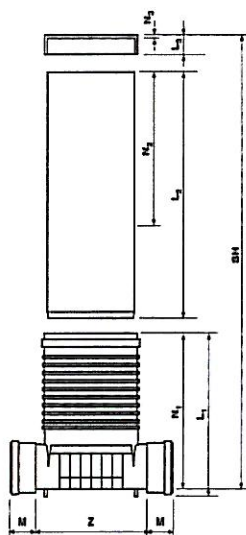
Schéma stavby šachty A 15
