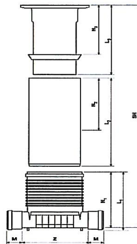
Schéma stavby šachty B 125/ D 400
